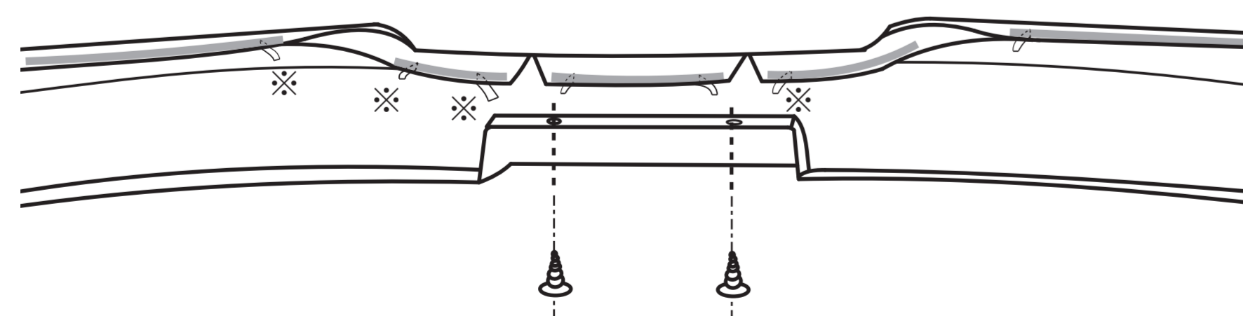
両面テープ (スポイラーの裏側)
